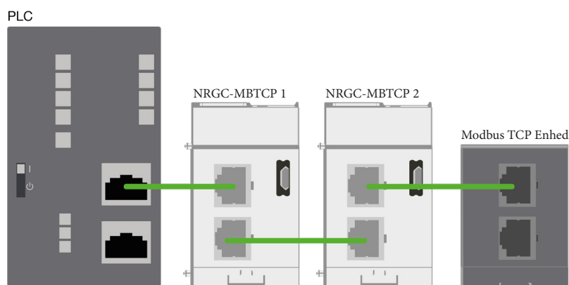
Figur. 3 Eksempel på en linjekonfiguration af NRGC-MBTCP med andre Modbus TCP-enheder og -kontrolenheder
