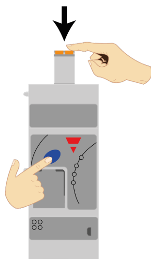
Fig. 1 Tenere premuto il pulsante blu mentre si accende NRG-MBTCP
