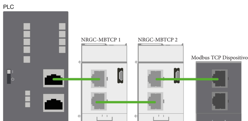
Fig. 3 Esempio di una configurazione in linea di NRGC-MBTCP con altri dispositivi e controllore in Modbus TCP
